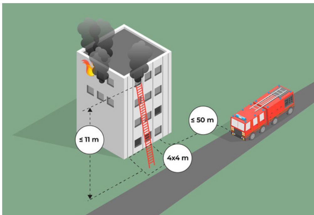
Figur 2: Illustration av de krav som behöver uppnås för att kunna tillgodoräkna utrymning med hjälp av räddningstjänstens bärbara stegar.
