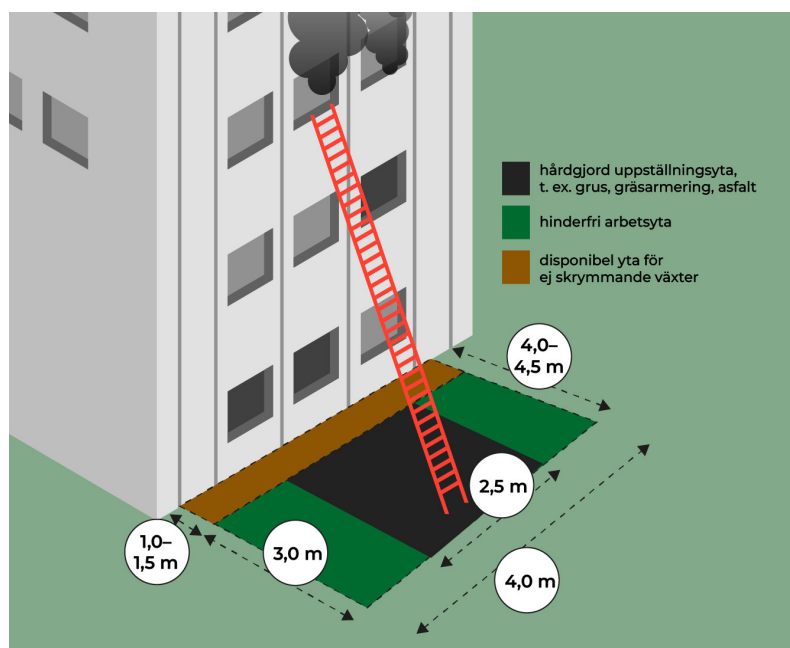
Figur 3: Illustration av utformningen av en uppställningsplats för bärbara stegar.
