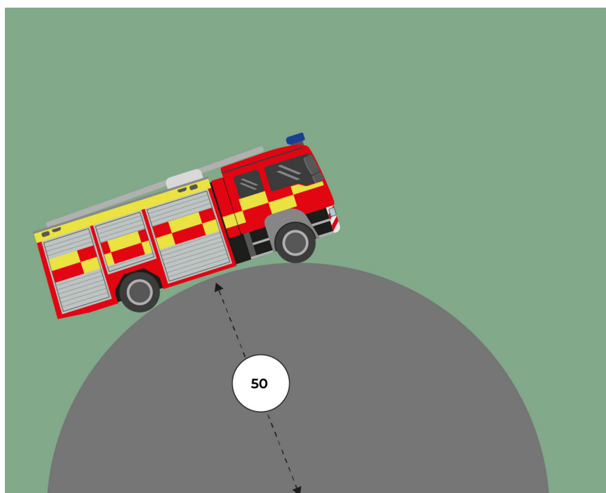
Figur 4: illustration på vad som avses med vertikalradie på > 50 \text{ m} .
